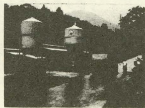
飼料バラ取りタンクとタンク車
